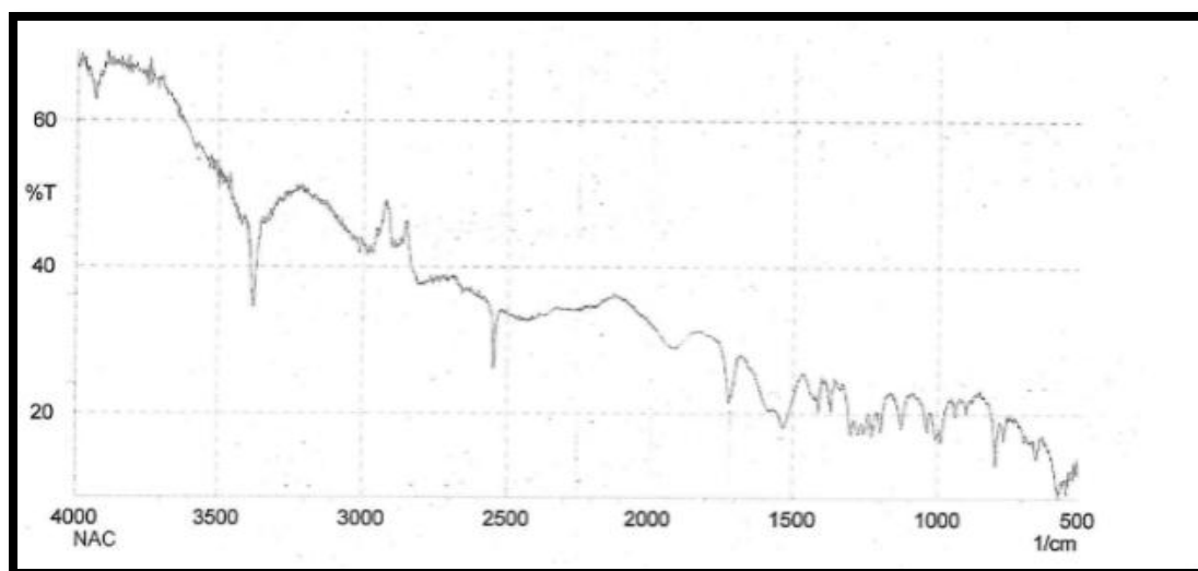
Fig no 1: IR Spectra of API.
